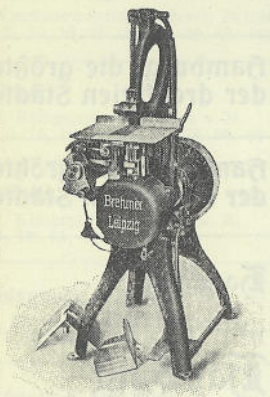
Broschüren- Drahtheftmaschine „Universal“ Nr. 7 1 / 2 bis 23 mm Dicke heftend
